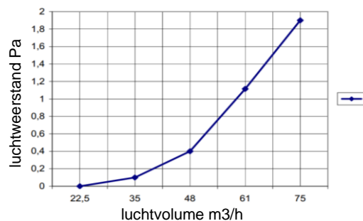
luchtweerstand aanslui. wand / vloer 2x75 artikel nr.7064
