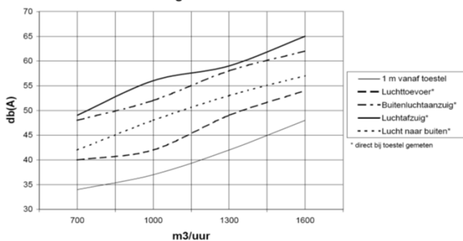
Geluidmeting KB1600CVK
