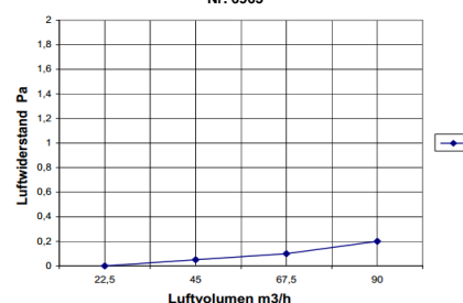
Luftwiderstand Anschl. Wand/Decke 305/102 4x50 Artikel Nr. 6965
