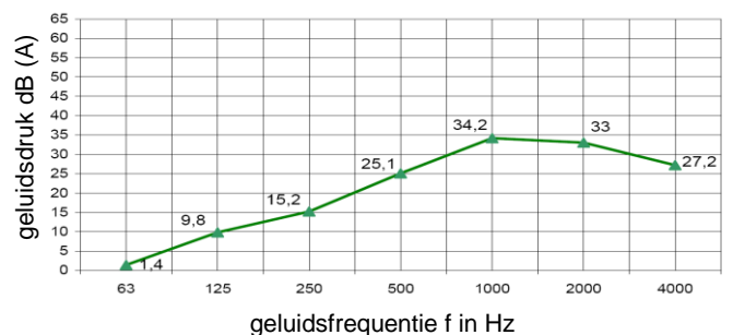
Geluidsdemping EuroAir luchtverdeler met geluiddemper
