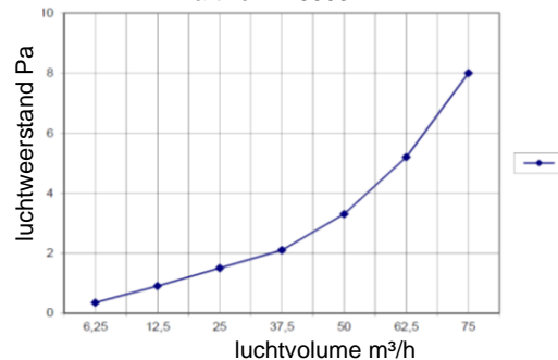
luchtweerstand hoekverloopstuk 125/2x75 artikel nr. 5593
