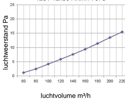
Luchtweerstand verdeler met int. Demper 125 / 12x50 Art.nr. 7078
