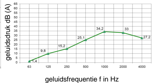
Geluidsdemping EuroAir luchtverdeler met geluiddemper
