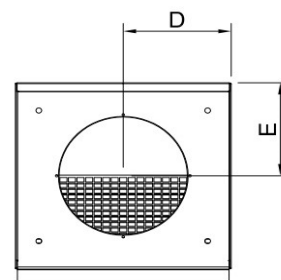
Rückansicht
