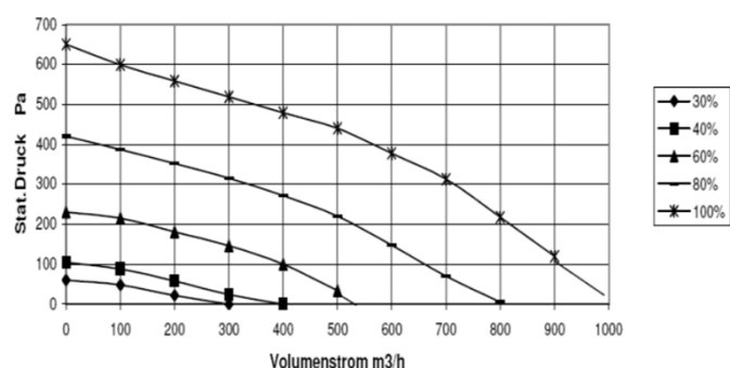
Volumenstrom EuroAir Klimabox 800
