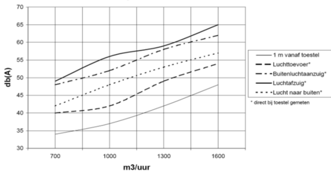
Geluidmeting KB1600CVK
