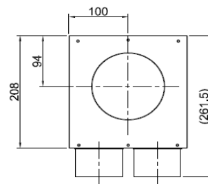
bovenaanzicht
