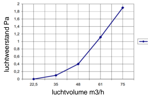
luchtweerstand aanslui. wand / vloer 3x50 artikel nr.7063
