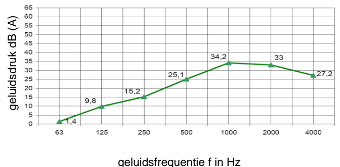
Geluidsdemping EuroAir luchtverdeler met geluiddemper
