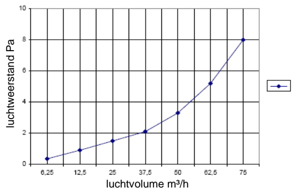
luchtweerstand hoekverloopstuk 125/2x75 artikel nr. 6955
